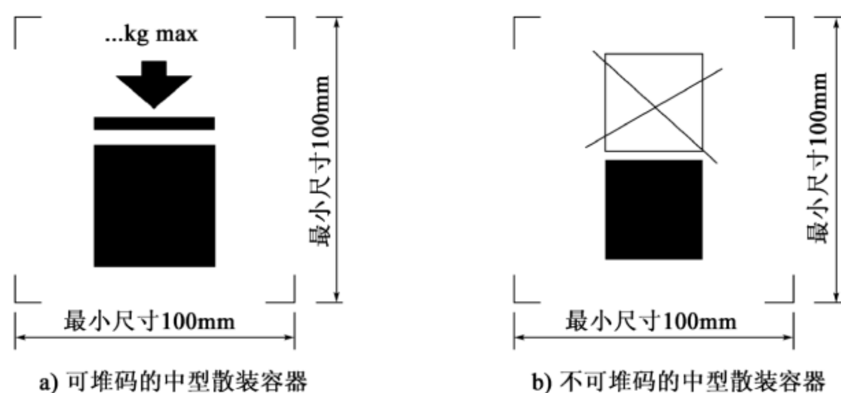
图 B.1 最大允许堆码负荷标记
